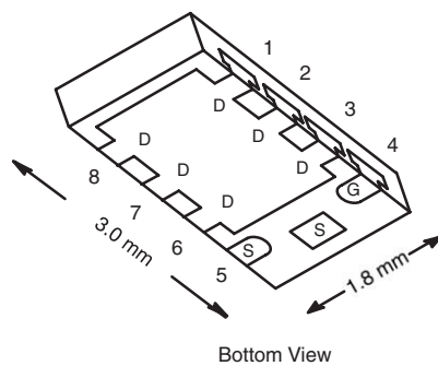
PowerPAK ChipFET Single
